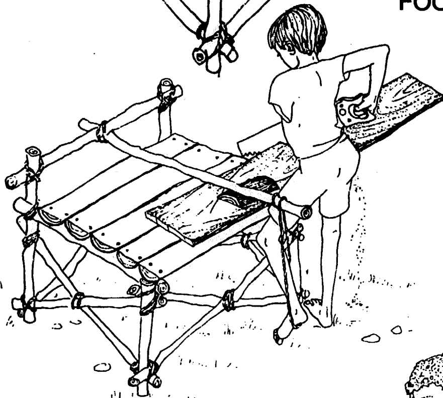
FOOT VICE
