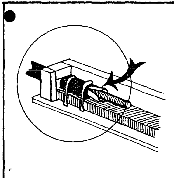
18 On glisse une autre bague Teflon entre le tube pivot et la tige de commande.
