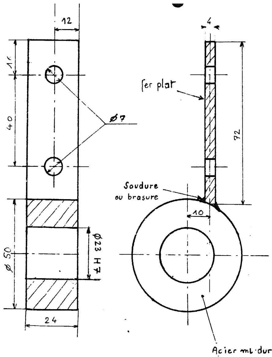
1 BIELLE
