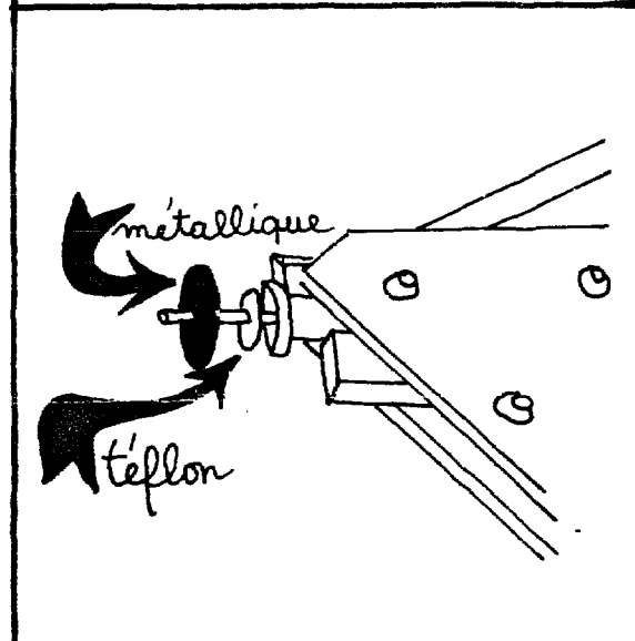
21 On met en place une rondelle Teflon et une rondelle métal
