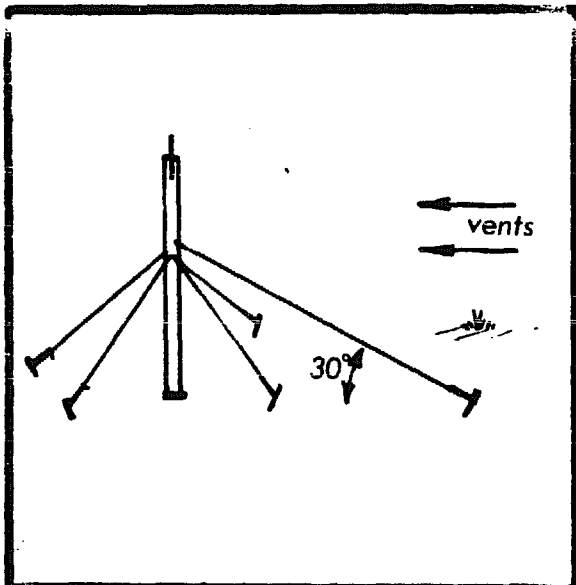
10 On place de cette manière 5 haubans.
