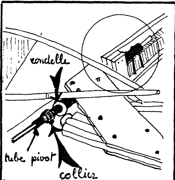
17 avec une rondelle et un collier serré sur un bourrelet de cuir enroulé autour du tube pivot.
