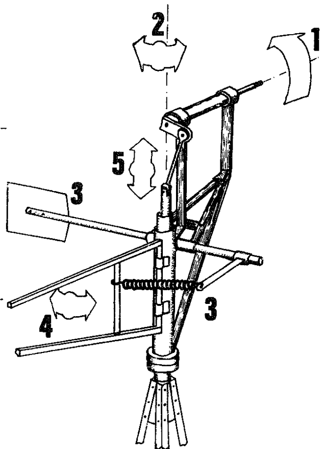
TÊTE D'EOLIENNE MULTIPALE : SES FONCTIONS
