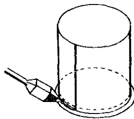
8. Mise en place et soudage du fond
